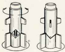
Verriegelung der Spulen Locking of spools Verrouillage des bobines Bloccaggio delle bobine
